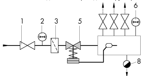
Рис. 3.2. Подключение трубки на распределителе
