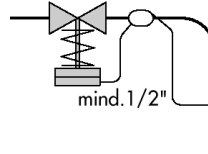
Рис.3.3 Подключение ниже середины фланца клапана
