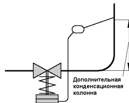
Рис. 3.4. Подключение выше середины фланца клапана
